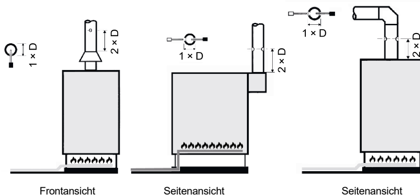
Abbildung 4: Messort bei atmosphärischen Gasheizgeräten mit Strömungssicherung
