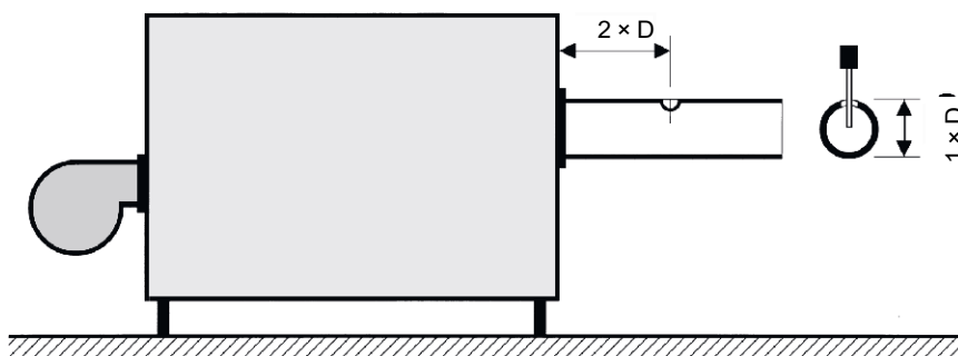
Abbildung 1: Messort bei Abgasrohr mit genügend langer gerader Strecke vor einem Rohrbogen (Öl-, Gas- und Holzfeuerungen)
