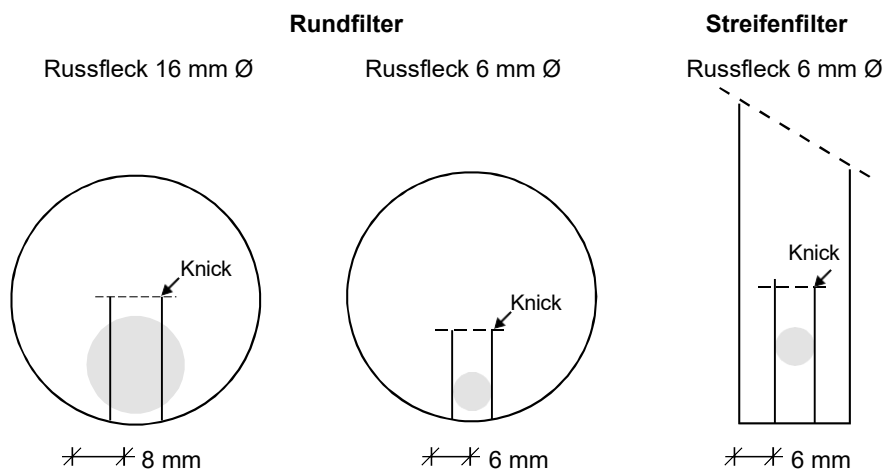
Abbildung 5: Streifen in das Filterpapier schneiden
