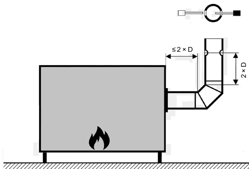
Abbildung 4: Messort bei atmosphärischen Gasheizgeräten mit Strömungssicherung
