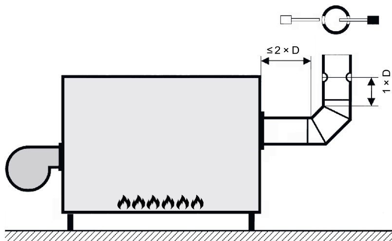
Abbildung 2: Messort bei Abgasrohr, das vor einem Rohrbogen keine genügend lange gerade Strecke aufweist (Öl- und Gasfeuerungen)
